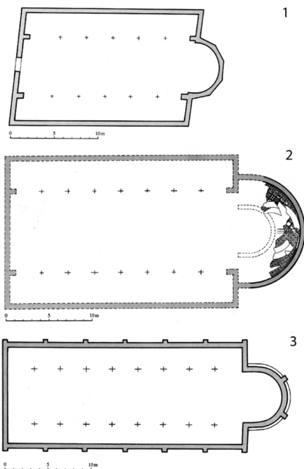
Сл. 5 1) Нин, базилика Св. Марије, V в. 2) Острво Паг, Новаља, базилика Св. Марије, V в. 3) Базилика на Старом гробљу, V в. Планови према П. Вежићу.
