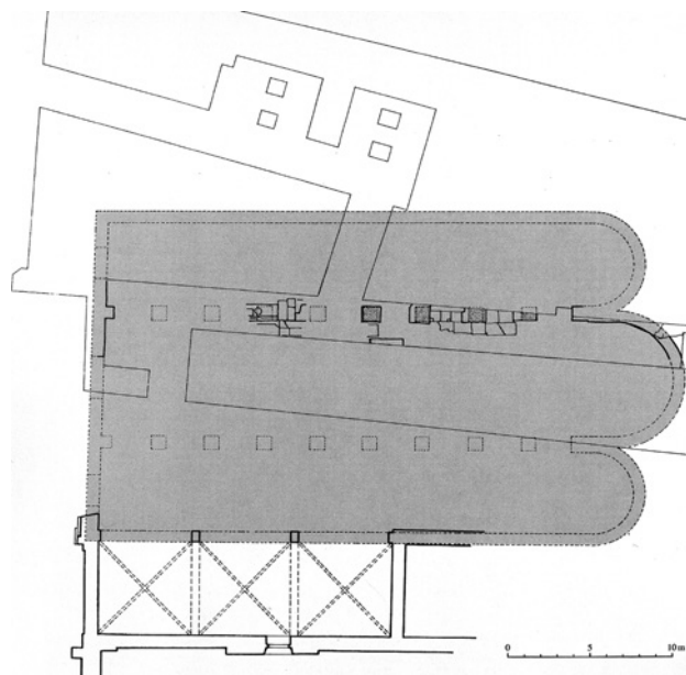
Сл. 9 Задар, базилика Св. Марије Велике, V в. План према П. Вежићу.
