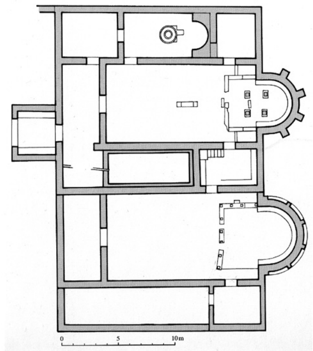
Сл. 15 Двојне базиликеу Срими, IV – VI в. План према П. Вежићу.
