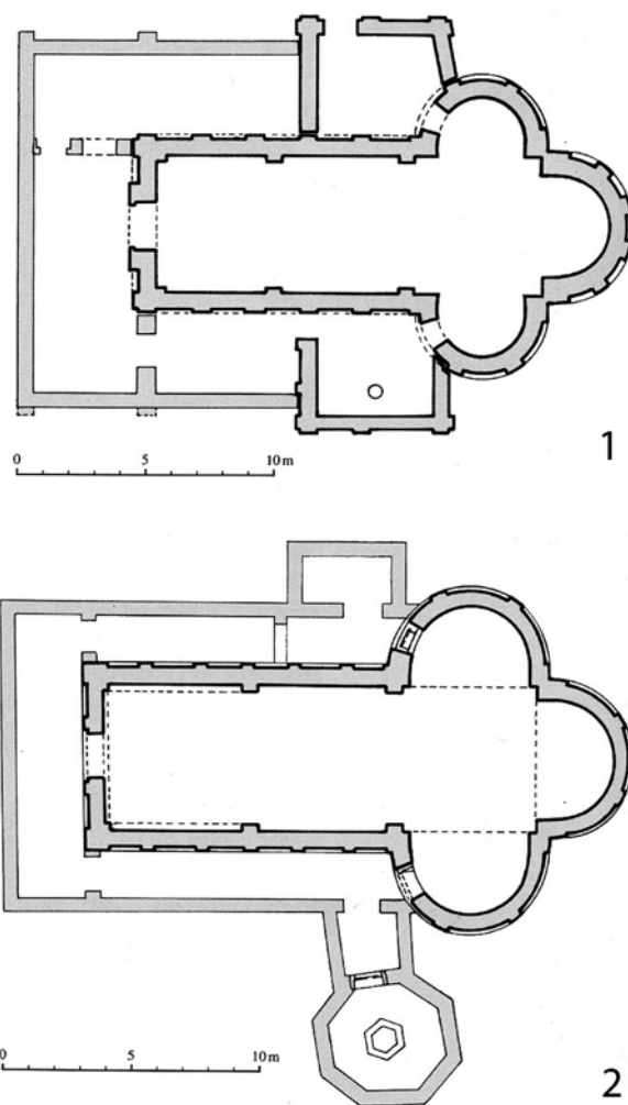
Сл. 13 1) Меморија у Билицама, V–VIв. 2) Црква Св. Мартина у Придрази, IV – VI в. Планови према П. Вежићу.
