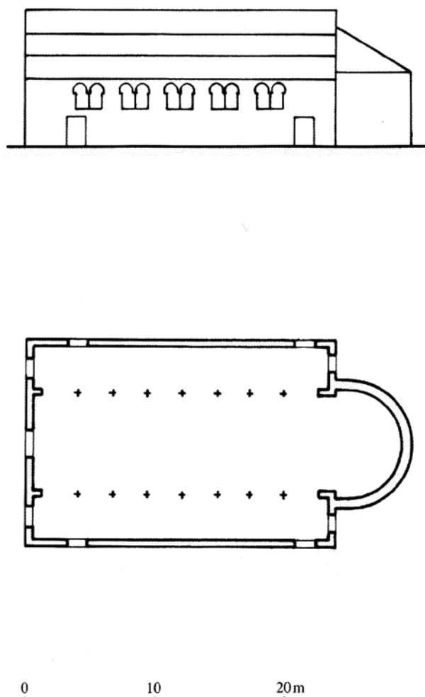
Сл. 4 Задар. Базилика Св. Томе, VI в. План и бочна фасада према П. Вежићу.
