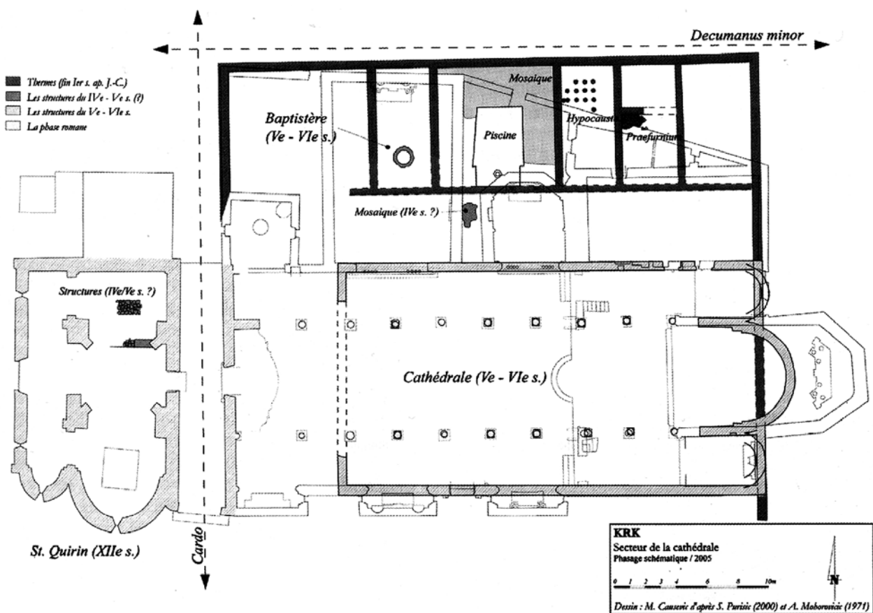
Сл. 7 Острво Крк, г. Крк, базилика Св. Марије, V–XIIIвв. План према С. Пуршићу и А. Мохоровићу. Fig. 7 Island of Krk, city of Krk, St Mary Cathedral, V c. Plan according to C. Purišić and A. Mohorovičić.
