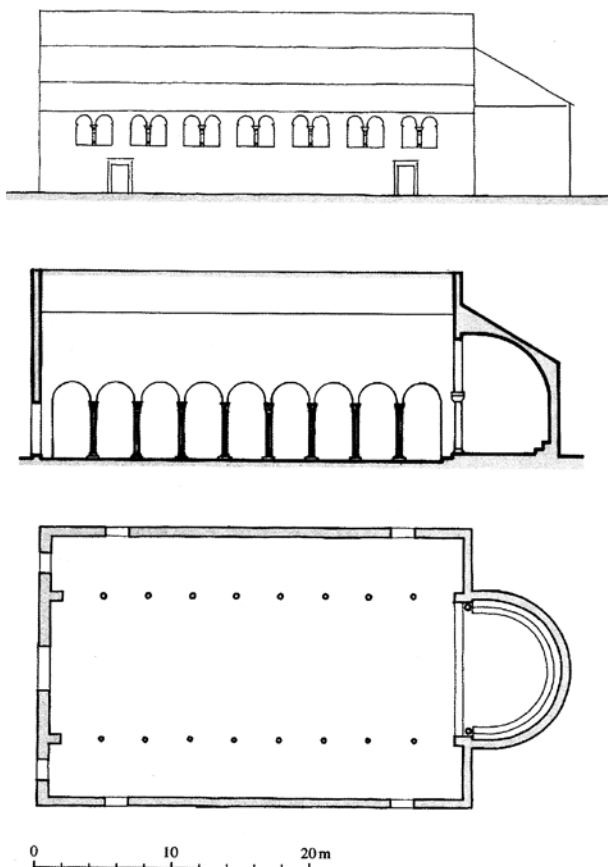
Сл. 3 Задар. Базилика Св. Стефана, V в. Бочна фасада, подужни пресек и план према П. Вежићу.
