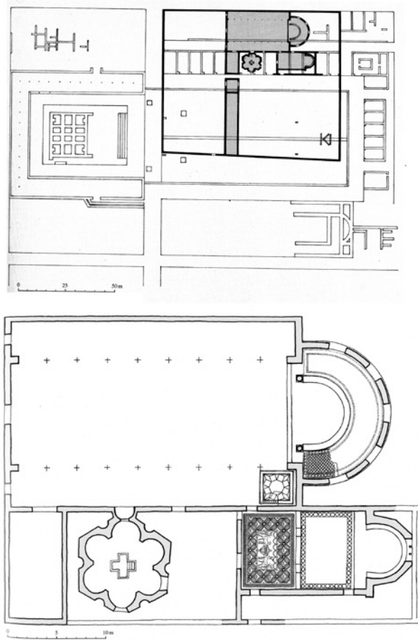
Сл. 1 Задар. План епископског комплекса и базилике IV-V в. Према П. Вежићу.
