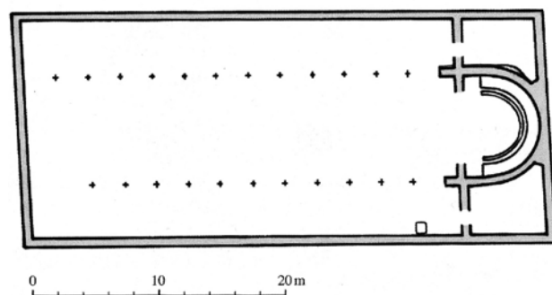
Сл. 10 Задар, базилика Св. Јована Крститеља на гробљу, V в. План према П. Вежићу.
