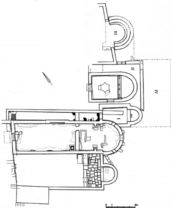
Сл. 8 Острво Црес, г. Осор, базилика Св. Марије, V в. Савремени план према М. Шиљак и М. Чаушевић.
